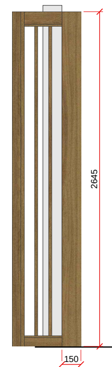
DIVISÓRIA RIPADA - LATERAL - ESC. 1:30
