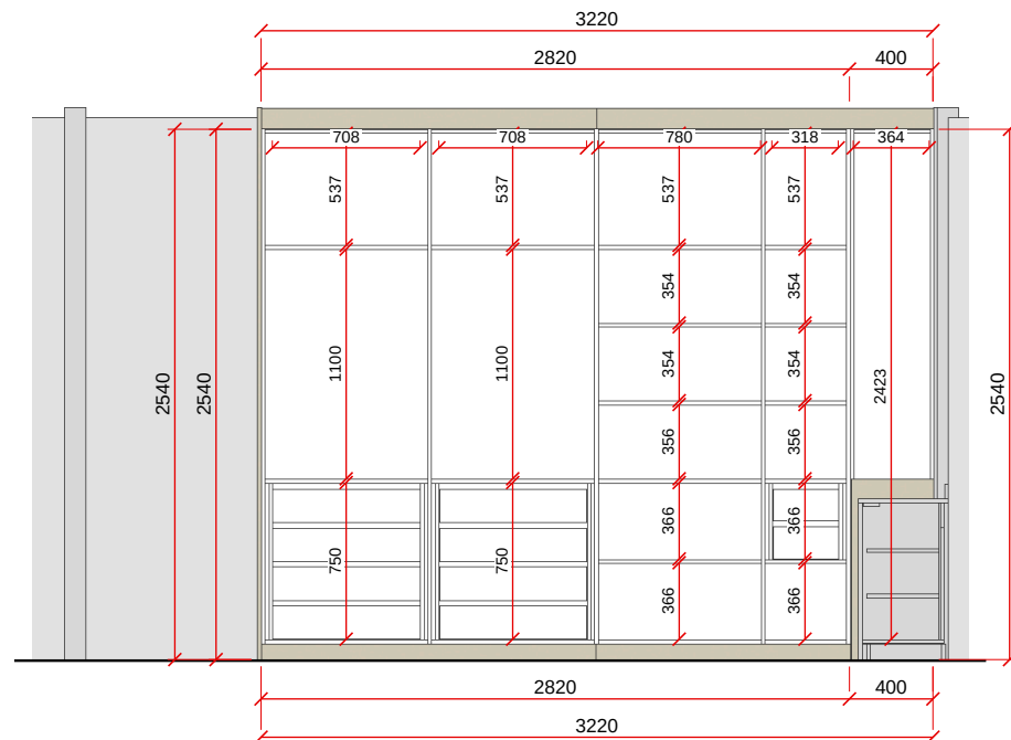
VISTA A - ESC. 1:40
