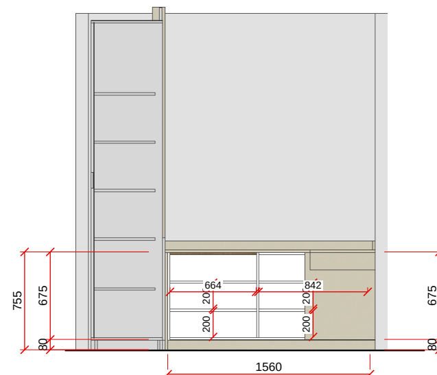
VISTA B - ESC. 1:40
