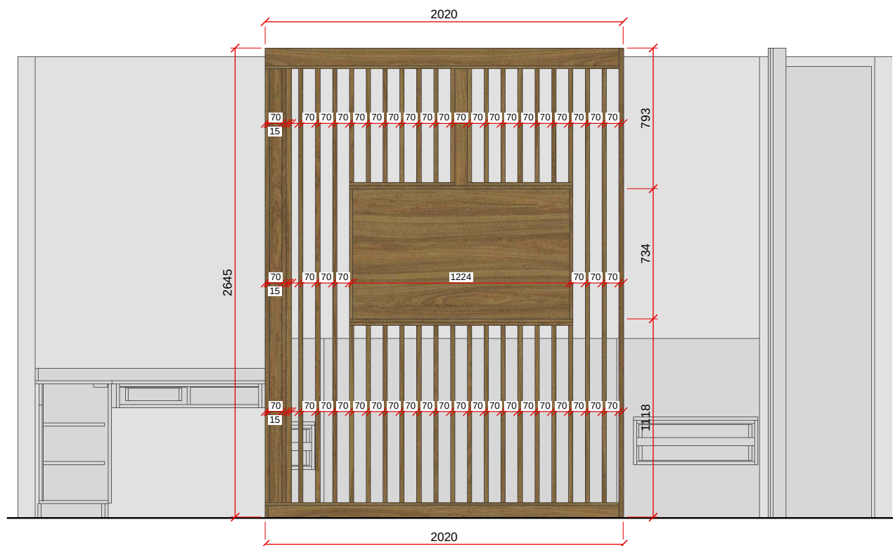
DIVISÓRIA RIPADA - ESC. 1:30
