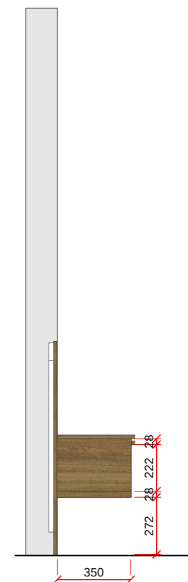
VISTA C - LATERAL - ESC. 1:25
